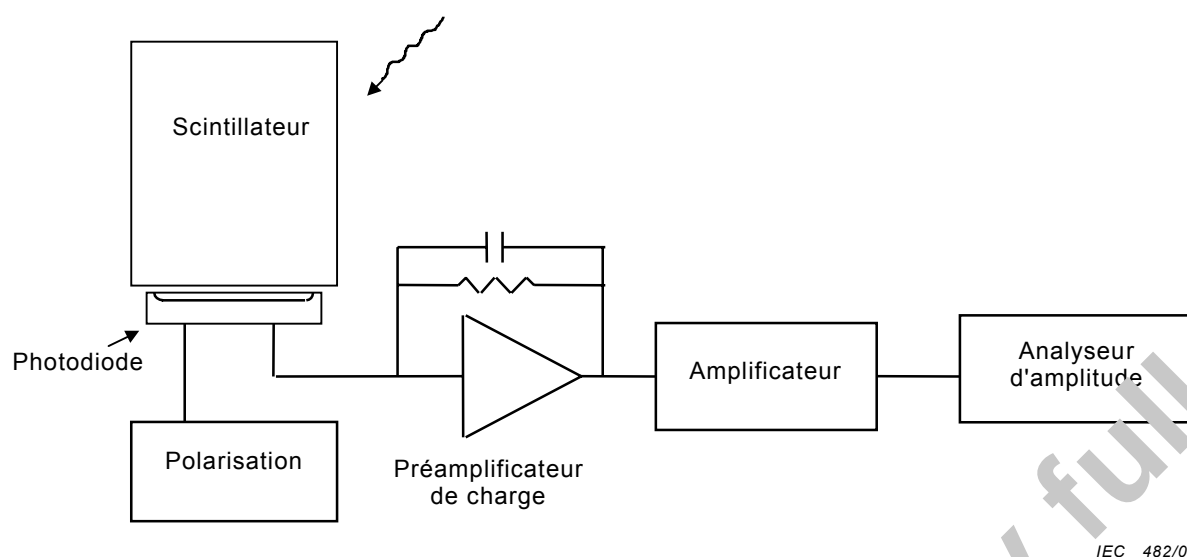
Figure 1 – Schéma d'un système avec détecteur à scintillation à photodiode
